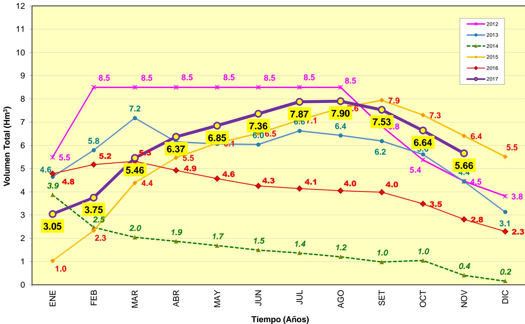
REGISTRO DE VOLÚMENES HISTÓRICOS DE LA REPRESA PAUCARANI 2012 AL 30 DE NOVIEMBRE DEL 2017
